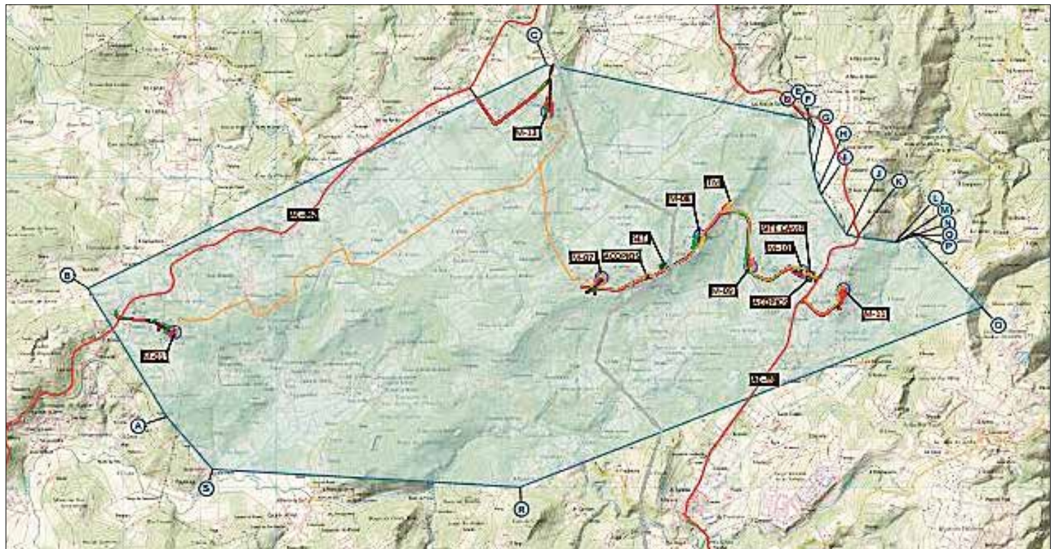
Poligonal que delimita o actual Parque Eólico Moeche, as posicións dos aerogeneradores, a torre meteorolóxica e a ubicación da subestación Moeche.
